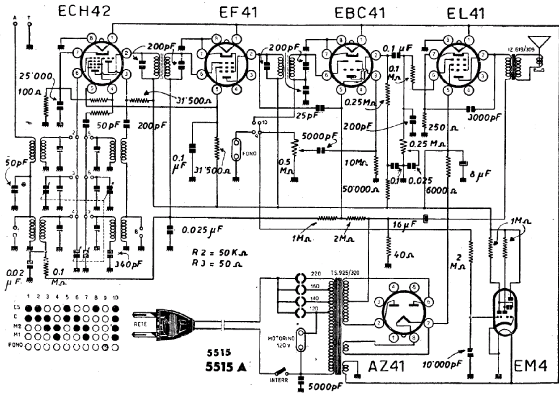
PHONOLA RADIO - Mod. 5515 e 5515 A - Medie e corte divise. MF. a 470 kc. Placca finale 350 V, schermo 250 V. Altre placche 250 V, schermi 85 V. Massimo negativo - 2 V. Consumo 40 W, uscita 4 W.
